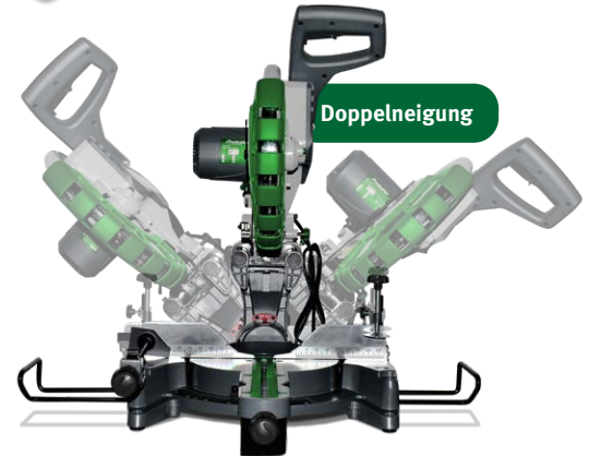
KGZ 305 E
