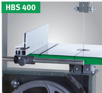
HBS 400 Sekundenschneller Umbau des Aluminium-Anschlags über Schnellspannhebel für Arbeiten mit flachem Anschlag
