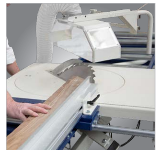
Sägeblattdrehung um bis zu 90°
