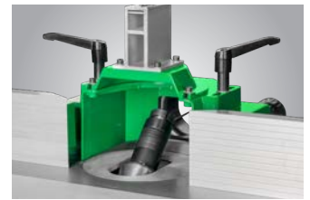
Nach hinten schwenkbare Frässpindel für optionalen Einsatz eines Vorschubapparates, ein Maximum an Sicherheit und ein sauberes Fräsbild
