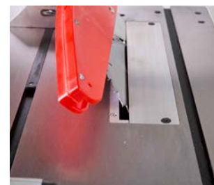
Sägeblattschwenkung von 90° bis -45° nach links
