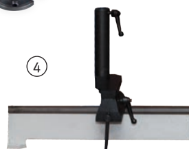
Massive Stahlkonstruktion nur für Handdrehselbänke mit drehbarem Spindelstock.
