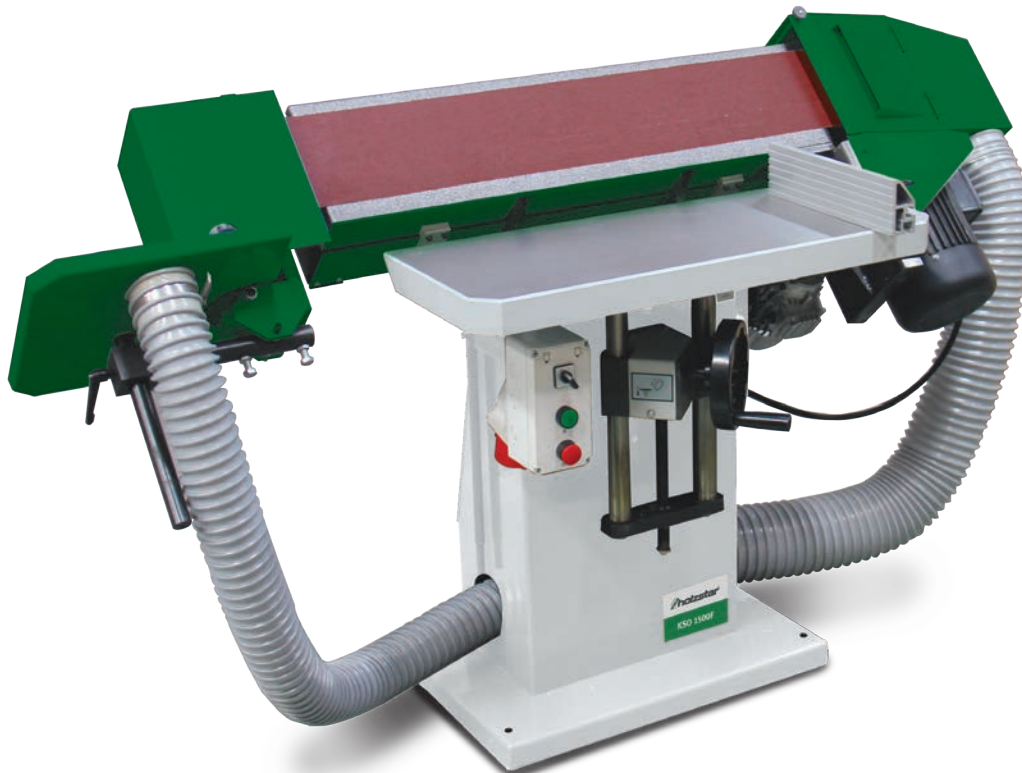
Höhenverstellbarer Zusatztisch mit Absaugung, zum Schleifen von Innenradien
