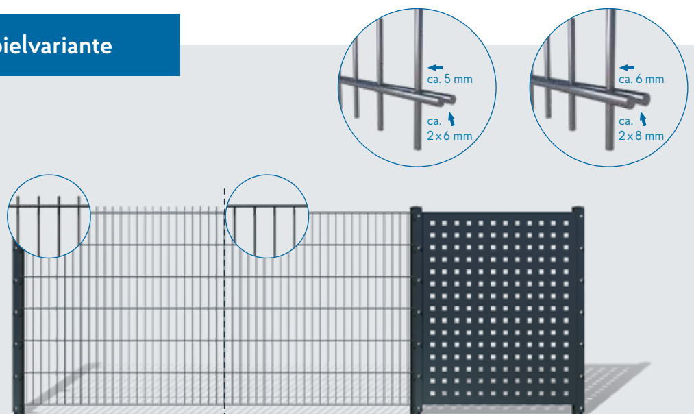
Doppelstabmatte mit Drahtüberstand / ohne Drahtüberstand / mit Loch-Designblech
