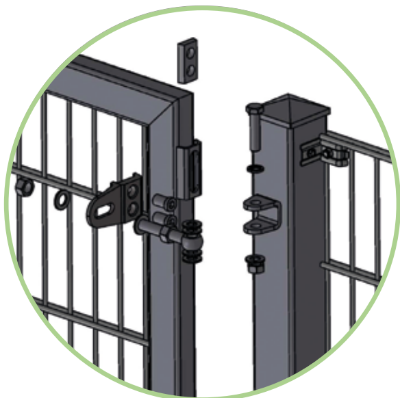
Torband:
