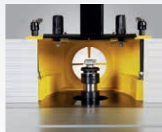
Frässpindel mit 80 mm Nutzlänge und 30 mm Durchmesser
